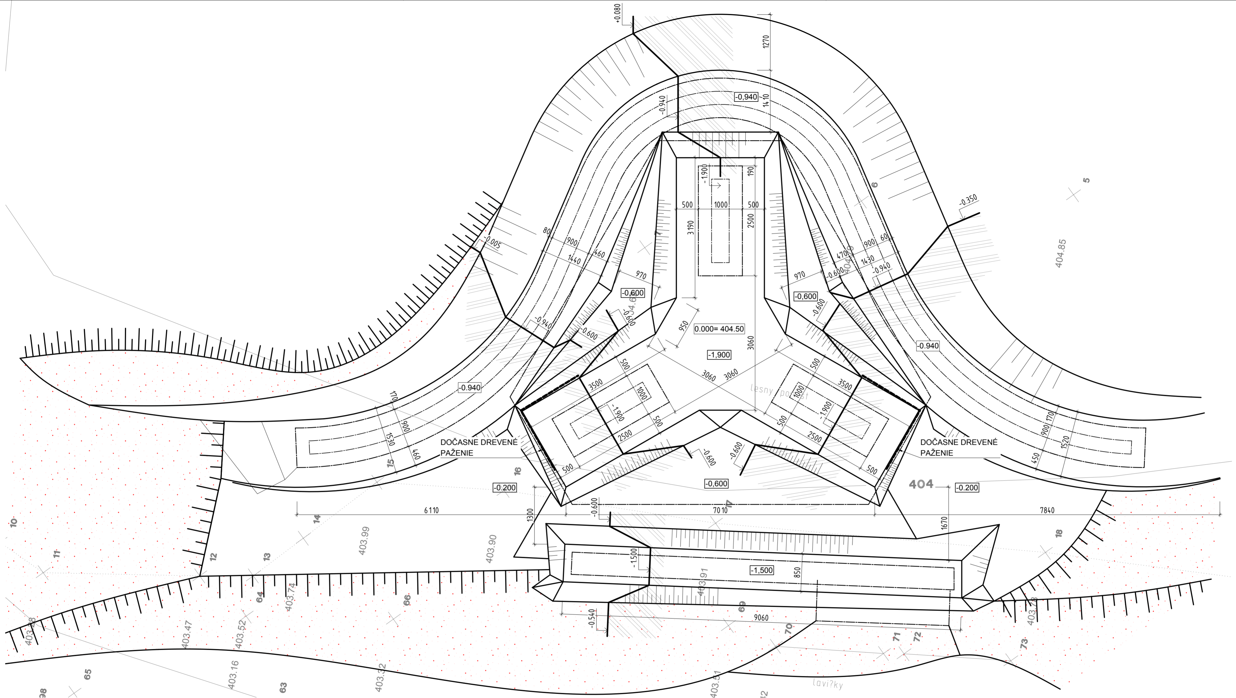
PODORYS VÝKOPOV A NÁSYPOV M 1:50
